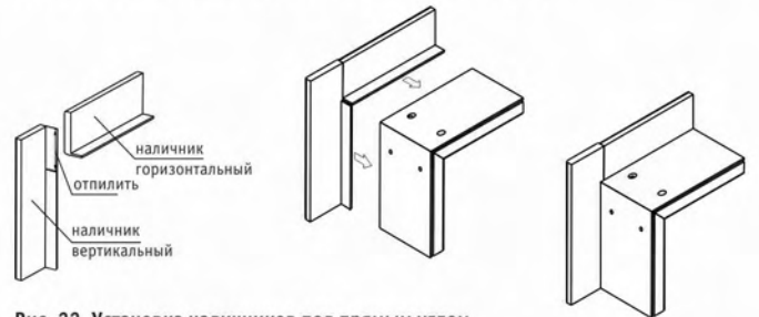
Рис. 22. Установка наличников под прямым углом.
